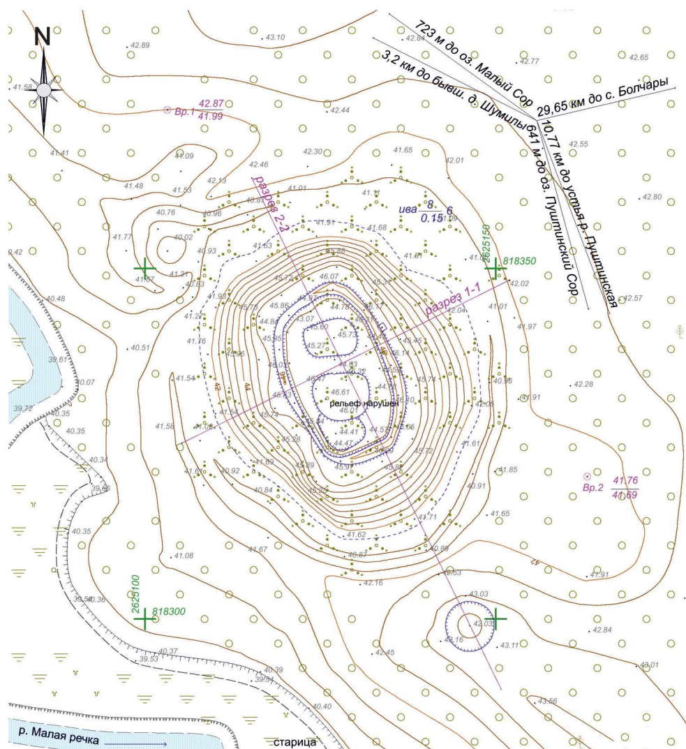
Рис. 3. Топографический план городка Вош-ега-вош
